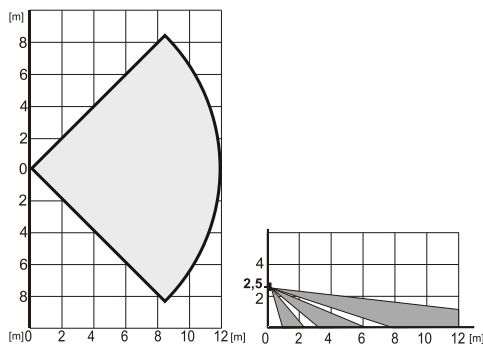
Abbildung 3: Diese Erkennungscharakteristiken gelten für die standardmäßige PIR-Immunität.
